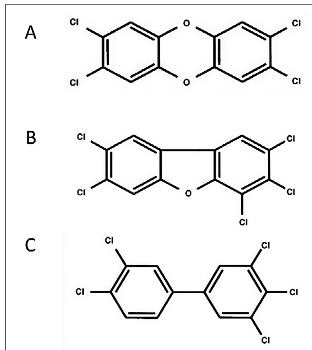
Rycina 1. Wzór strukturalny (A) dioksyny: 1,2,3,7,8-tetrachlorodibenzodoksyna, (B) furanu: 2,3,4,7,8-pentachlorodibenzofuran, (C) fenyly: 3,3',4,4',5-pentachlorobifenyl (PCB 126)
