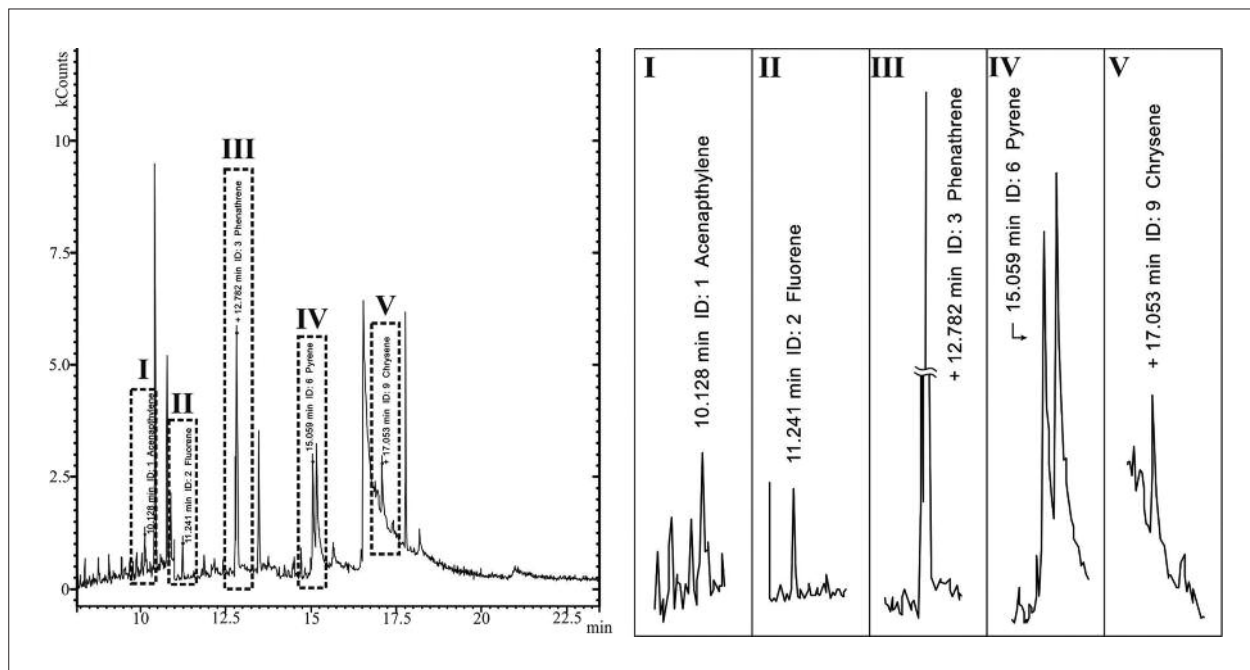
Ryc. 3. Chromatogram przedstawiający zawartość WWA w sokach drzewnych brzoźowych (acenaftylen, fluoren, fenantren, piren, chryzen)
